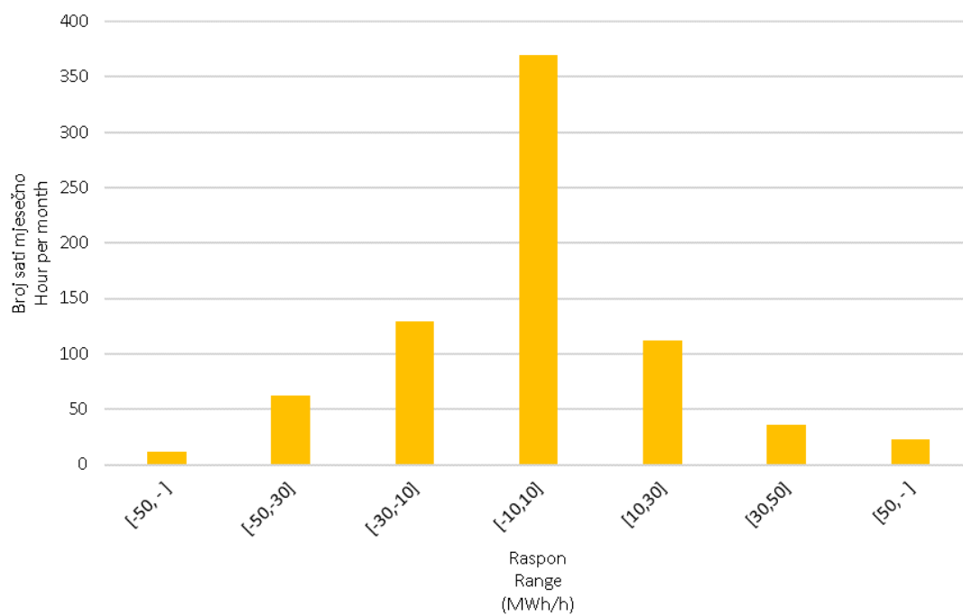
Slika 10 Statistička raspodjela satnih promjena proizvodnje VE u siječnju 2020. godine
