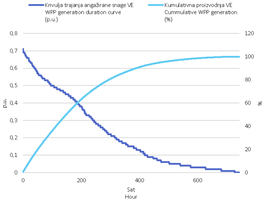
Slika 3 Krivulja trajanja angažirane snage svih VE i kumulativna proizvodnja VE u siječnju 2020. godine u jediničnim vrijednostima
