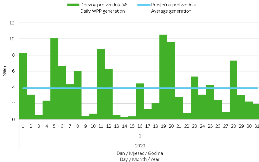
Slika 5 Dnevna proizvodnja svih vjetroelektrana u siječnju 2020. godine
