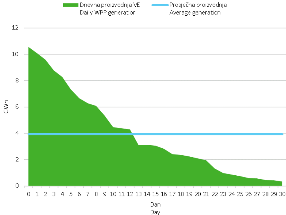
Slika 6 Krivulja trajanja dnevne proizvodnje vjetroelektrana u siječnju 2020. godine
