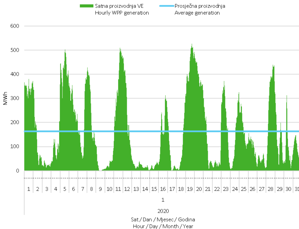
Slika 2 Satna proizvodnja svih vjetroelektrana u siječnju 2020. godine
