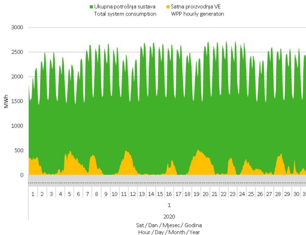
Slika 7 Usporedba satnog dijagrama opterećenja sustava i proizvodnje vjetroelektrana u siječnju 2020. godine
