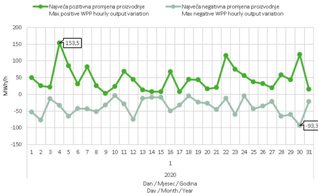
Slika 9 Maksimalna pozitivna i maksimalna negativna promjena satne proizvodnje VE u siječnju 2020. godine
