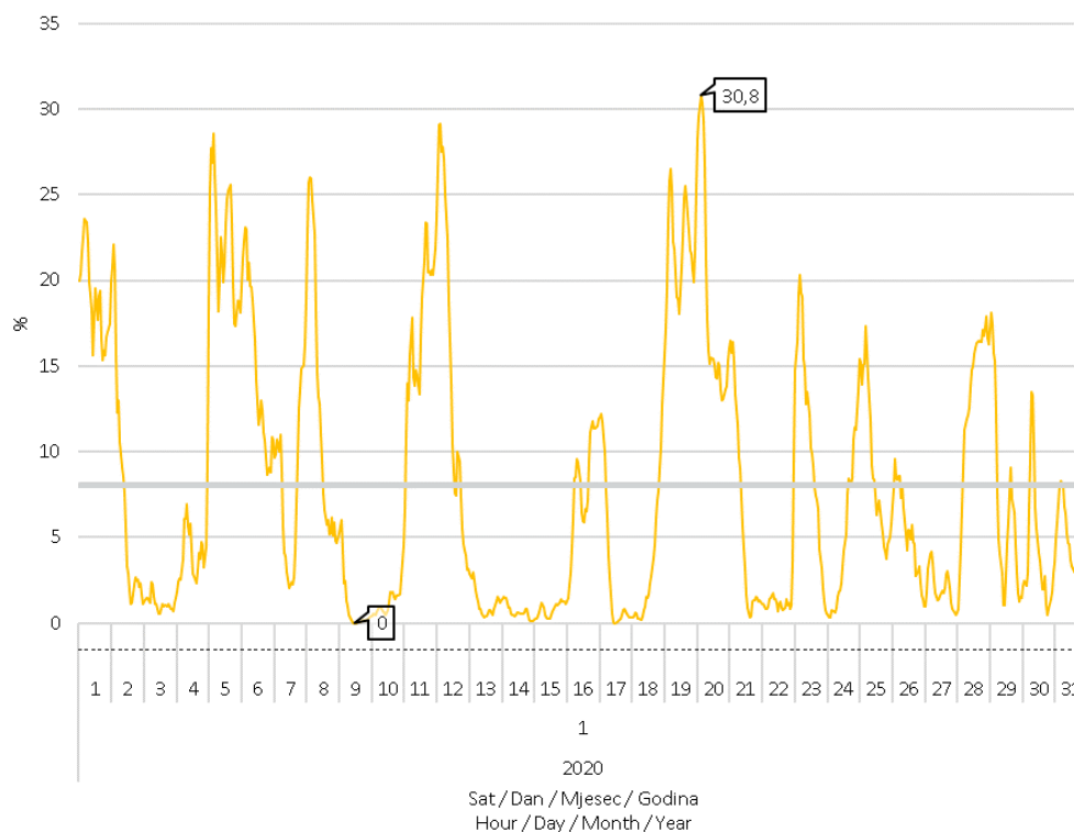
Slika 8 Udio proizvodnje vjetroelektrana u pokrivanju satnog opterećenja elektroenergetskog sustava u siječnju 2020. godine
